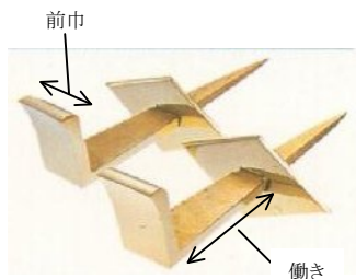
額受け金具
