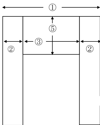
④ 三つ割り御簾 寸法の測り方
